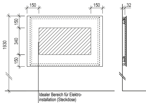
Maßskizze 24
