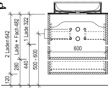
Maßskizze 1
