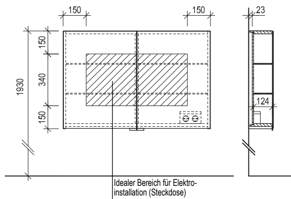
Maßskizze 25
